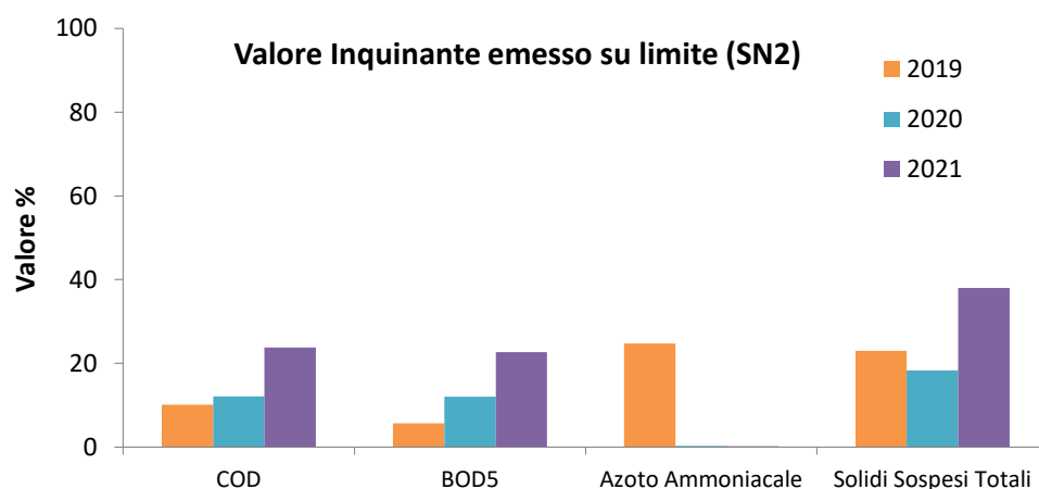
Figura 28 Andamento Indicatore "Posizionamento rispetto al limite" SN2
