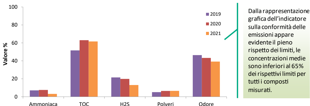
Figura 31 Andamento dell'indicatore "Posizionamento rispetto al Limite" – (media biofiltri E1, E2, E3, E4)
