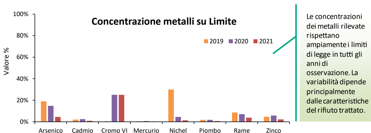
Figura 15 Andamento dell'indicatore "Posizionamento rispetto al limite"
