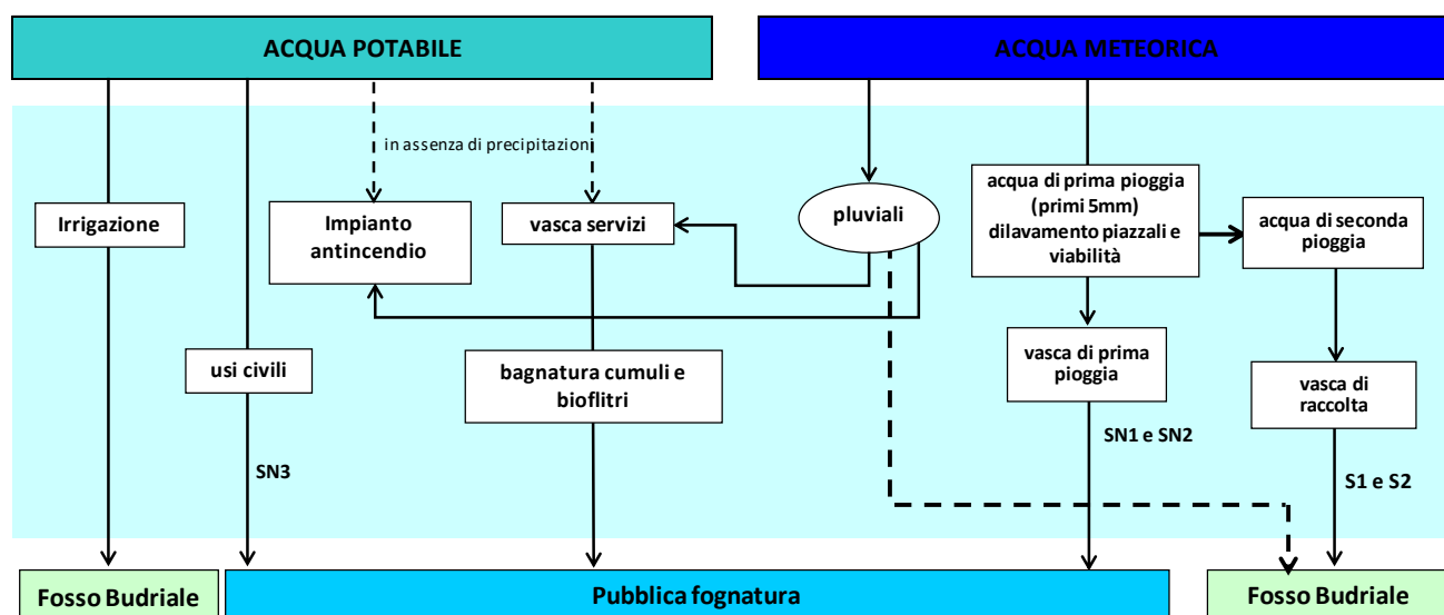
Figura 24 Ciclo idrico
