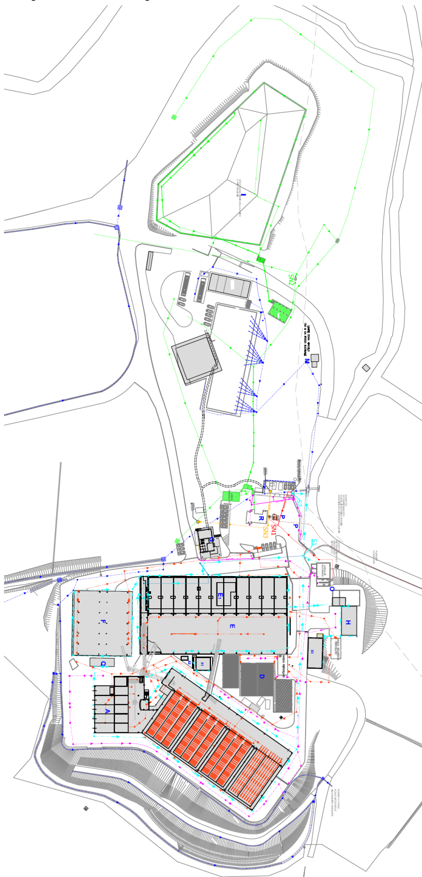
Figura 26 Planimetria degli scarichi idrici
