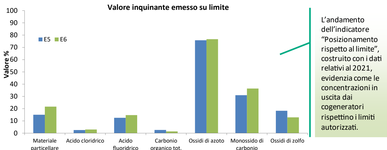
Figura 33 Andamento dell'indicatore "Posizionamento rispetto al Limite" – (emissioni E5 e E6)
