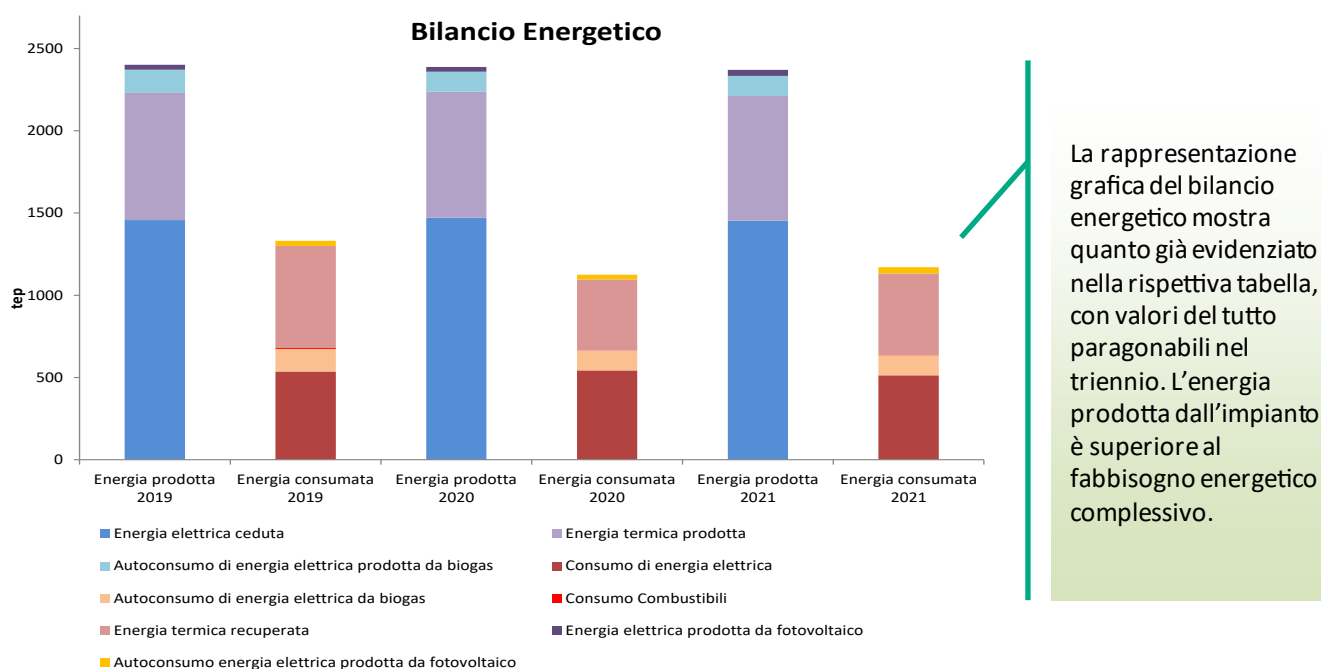
Figura 19 Bilancio energetico dell’impianto di compostaggio
