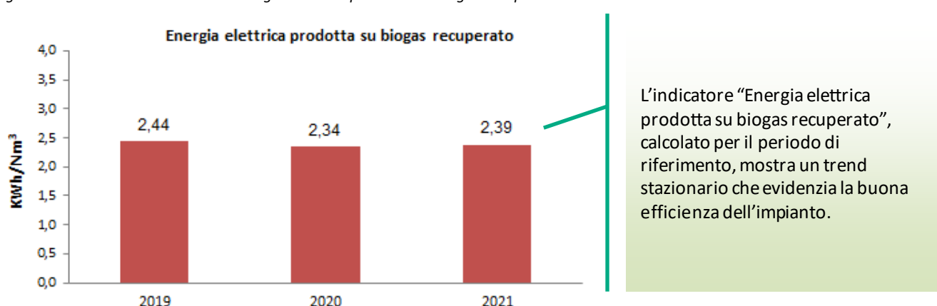
Figura 38 Andamento Indicatore "Energia elettrica prodotta su biogas recuperato"
